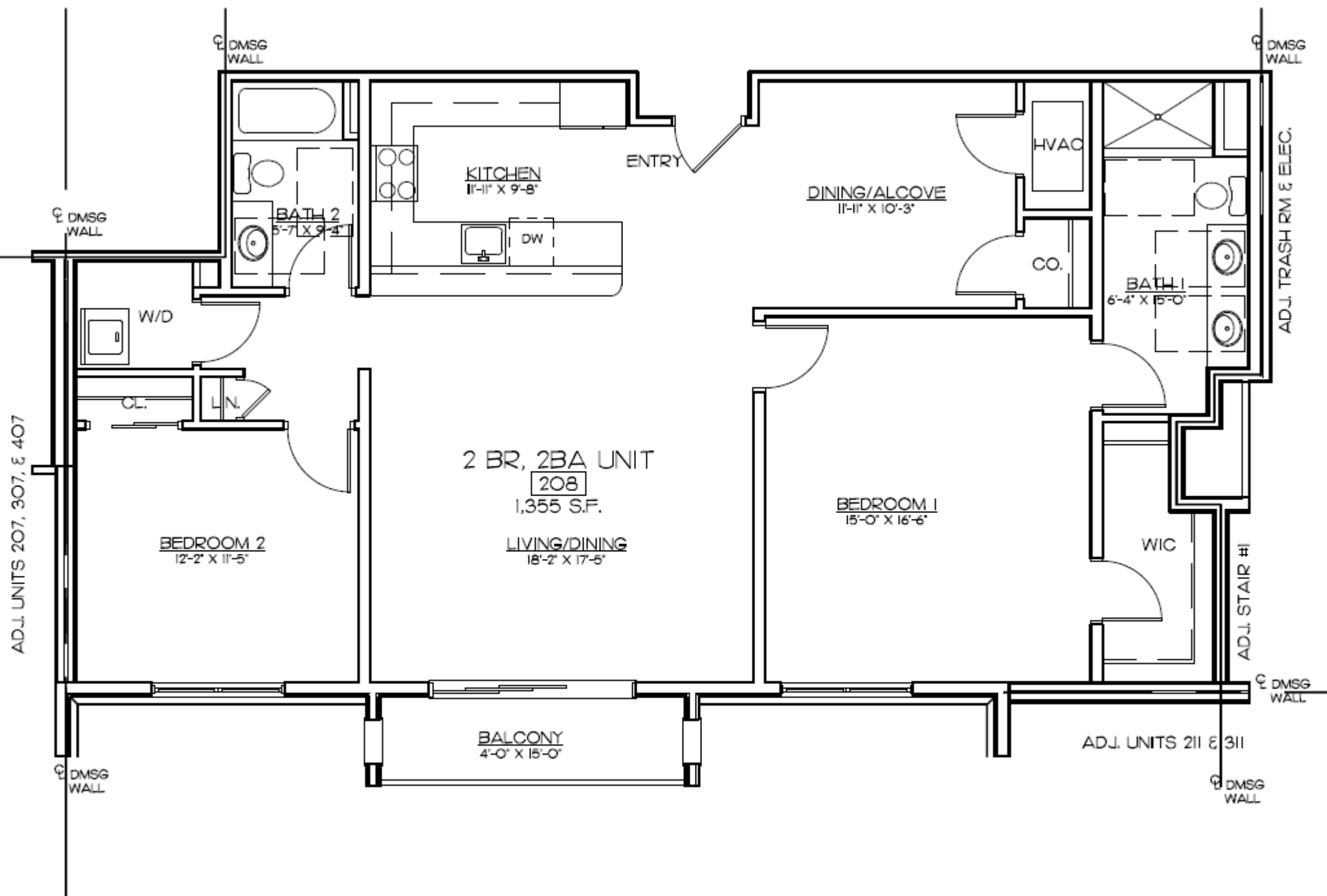
Units 208. 308. & 408 Scale: 1/8" = 1'-0"
